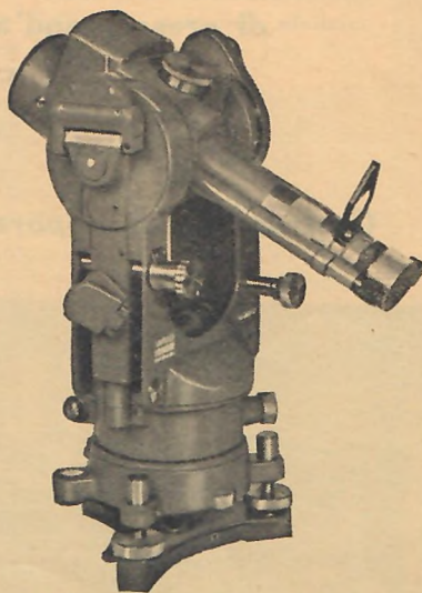
Tacheometro autoriduttore RDH per stadia orizzontale
